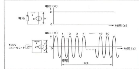
図 103 直流と交流による電圧の変化の違い
