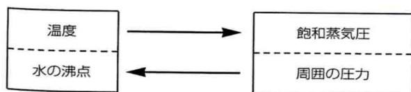
図5 温度と飽和蒸気圧の関係
