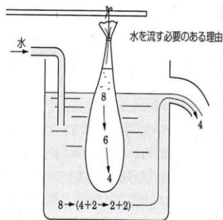
図 6 浸透圧の原理
