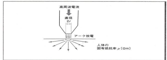
図 107 メス先部分での電気の流れ
