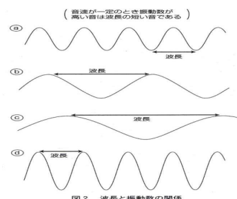
図 2 波長と振動数の関係
