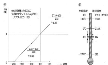
図4 セ氏温度と絶対温度の関係
